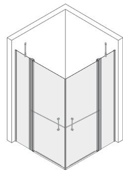
Eckeinstieg Drehtür 4-teilig TYP5171
